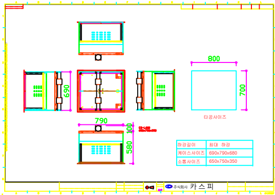
리프트(영사대). 전개도
